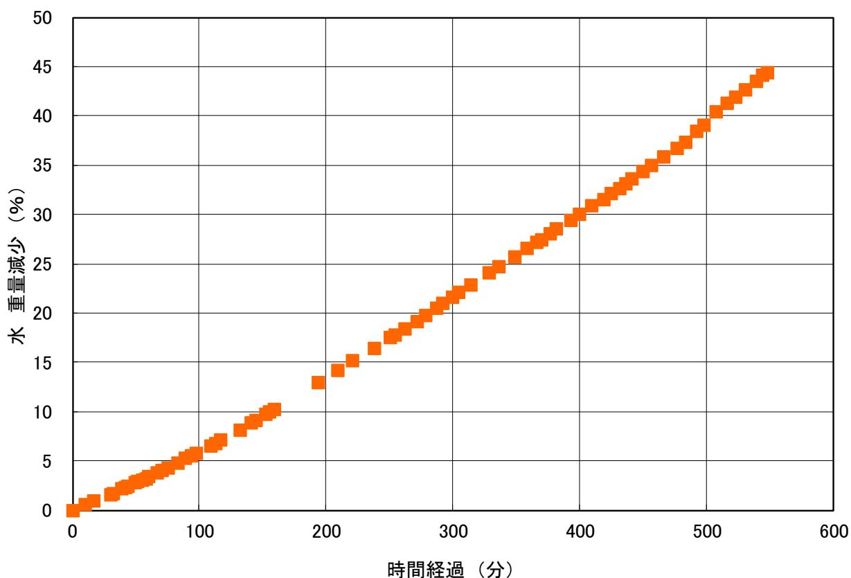
吸水性ポーラス金属体の水分徐放テスト (開始時の含水重量 5.37grを100%とする)
